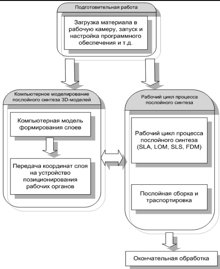
Рис. 2. Основные этапы методов послойного синтеза изделий
