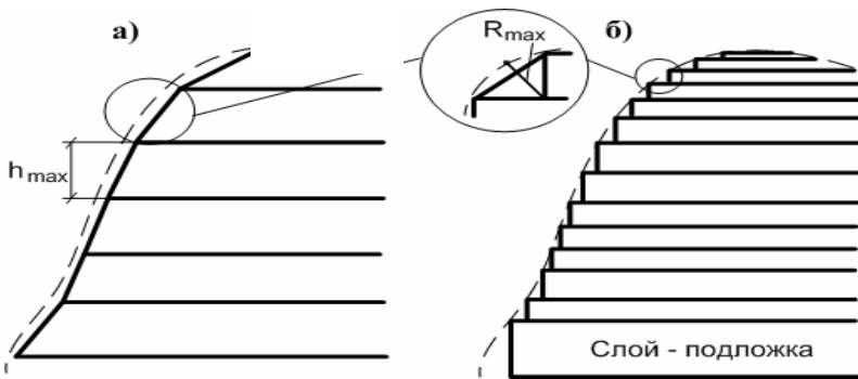
Рис. 4. Схема разбиения изделия на слои: для LOM- и FDM-процессов (а); для SLA- и SLS-процессов (б)
