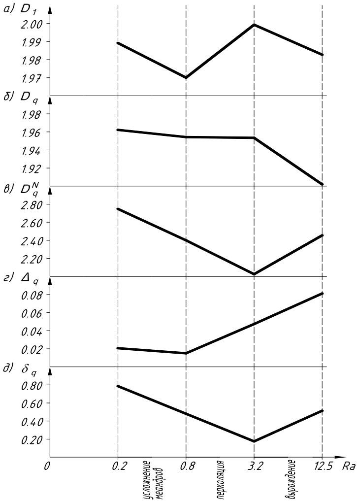
Рис. 8. Зависимости фрактальных характеристик покрытия, формируемого на основе с шероховатостью рельефа Ra : информационной размерности D_1 (а), экстремальных значений по управляющему параметру q размерности D_q (б), предельных значений D_q^N (в), степени упорядоченности \Delta_q (г) и степени разряженности \delta_q (д)
