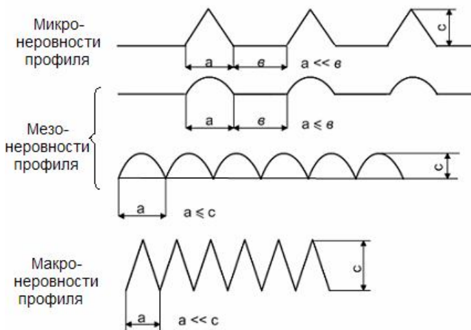
Рис. 5. Отклонения профиля границ слоев
