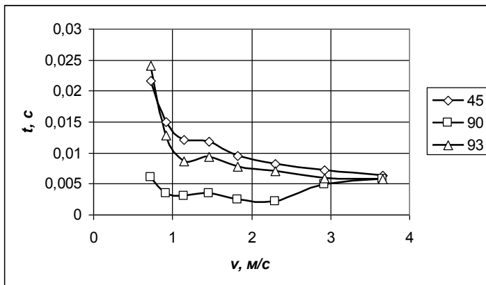
Рис. 9. Залежність збільшення фактичного часу тривалості вібрацій від швидкості різання
