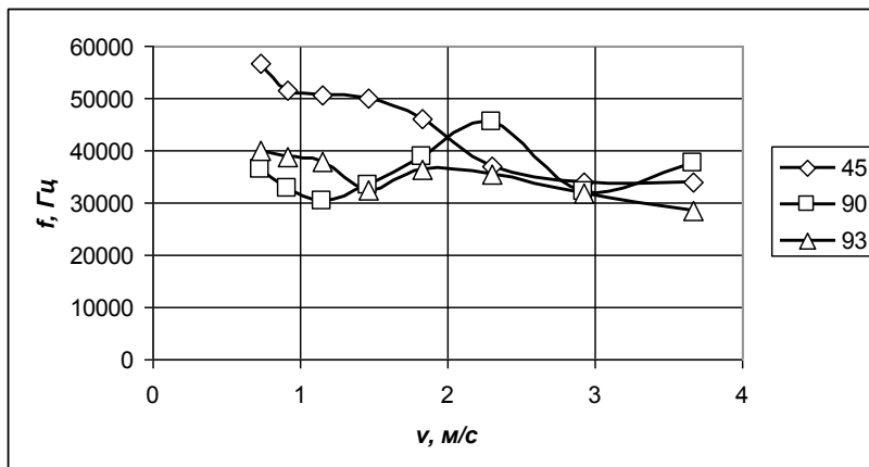
Рис. 6. Залежність частоти основної гармоніки вібросигналів від швидкості різання
