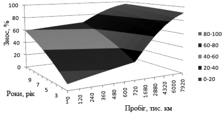
Рис. 2. Залежність фактичного зносу (%) автопоїздів Volvo від їх фактичного віку та пробігу
