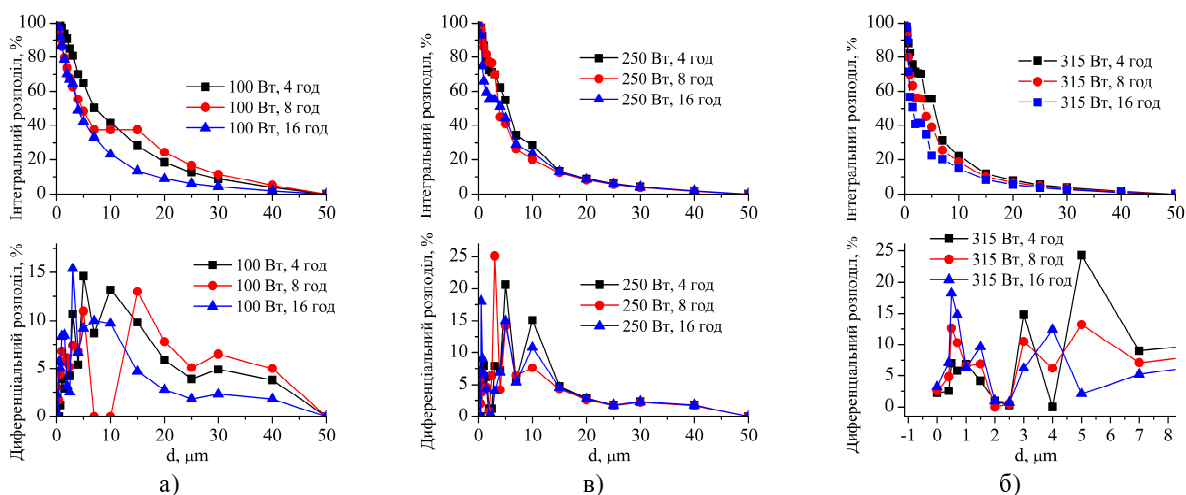
Рис. 3. Розподіл частинок НПГ після обробки ультразвуком за різних параметрах (час, потужність)
