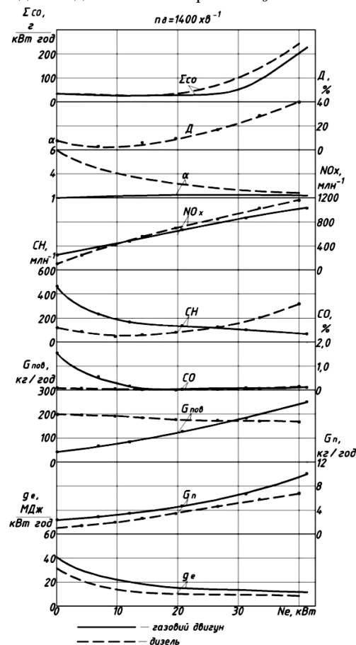
Рис. 2. Навантажувальна характеристика газового двигуна та дизеля при n_o = 1400 хв. -1
