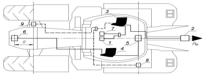
Рис. 3. Схема розташування обладнання на тракторі Fendt 936 Varіo: 1 – відеокамера; 2 – електронний динамометр; 3 – ноутбук для збереження результатів з відеокамери, GPS-навігатора, датчиків частоти обертання коліс та електронного динамометра; 4 – ноутбук для збереження результатів з акселерометрів; 5, 6 – акселерометри; 7 – GPS-навігатор; 8, 9 – датчики частоти обертання коліс; a = 0,75 м
