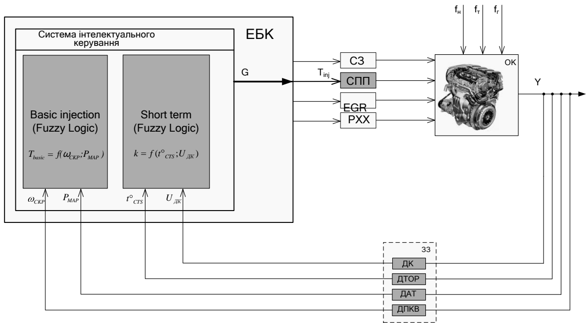
Рис. 5. Структурна схема системи інтелектуального керування подачею палива
