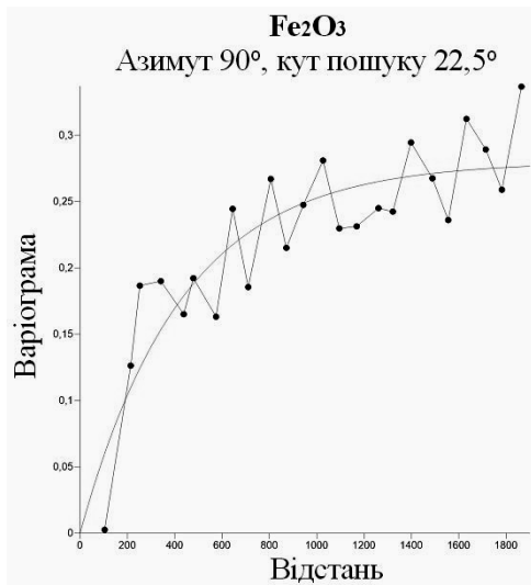
Рис. 2. Результат побудови варіограма та еліпсоїда анізотропії Fe 2 O 3
