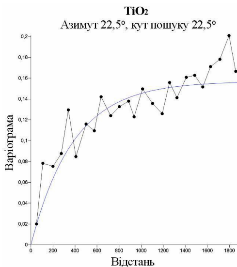
Рис. 3. Результат побудови варіограма та еліпсоїда анізотропії TiO 2
