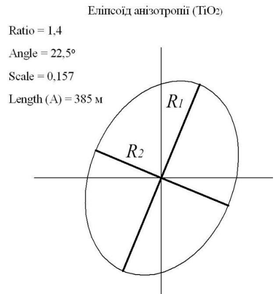
Рис. 3. Результат побудови варіограма та еліпсоїда анізотропії TiO 2
