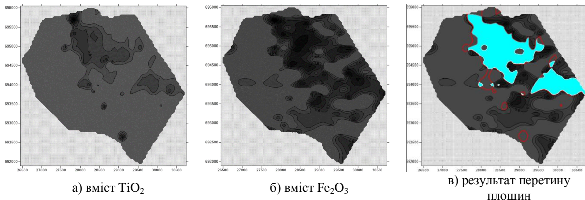
Рис. 9. Приклад визначення спільної зони за показниками якості для підрахунку об'єму каоліну сорту «КЭС-35» для виробництва електротермічного силуміну і ультрамарину із врахування коефіцієнта анізотропії
