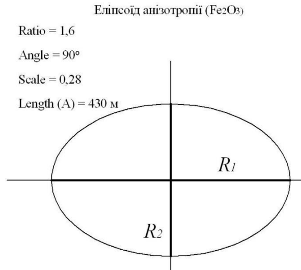
Рис. 2. Результат побудови варіограма та еліпсоїда анізотропії Fe 2 O 3
