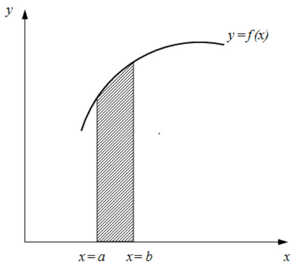
Рис. 5. Інтервал інтегрування [a, b]
