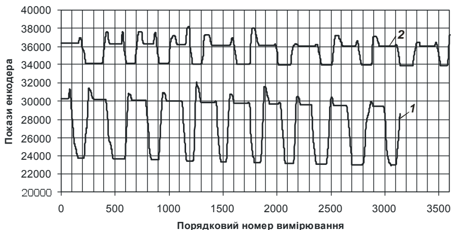
Рис. 2. Графіки часових залежностей серії вимірювань 1 — кінцева міра 60 мм; 2 — кінцева міра 20 мм
