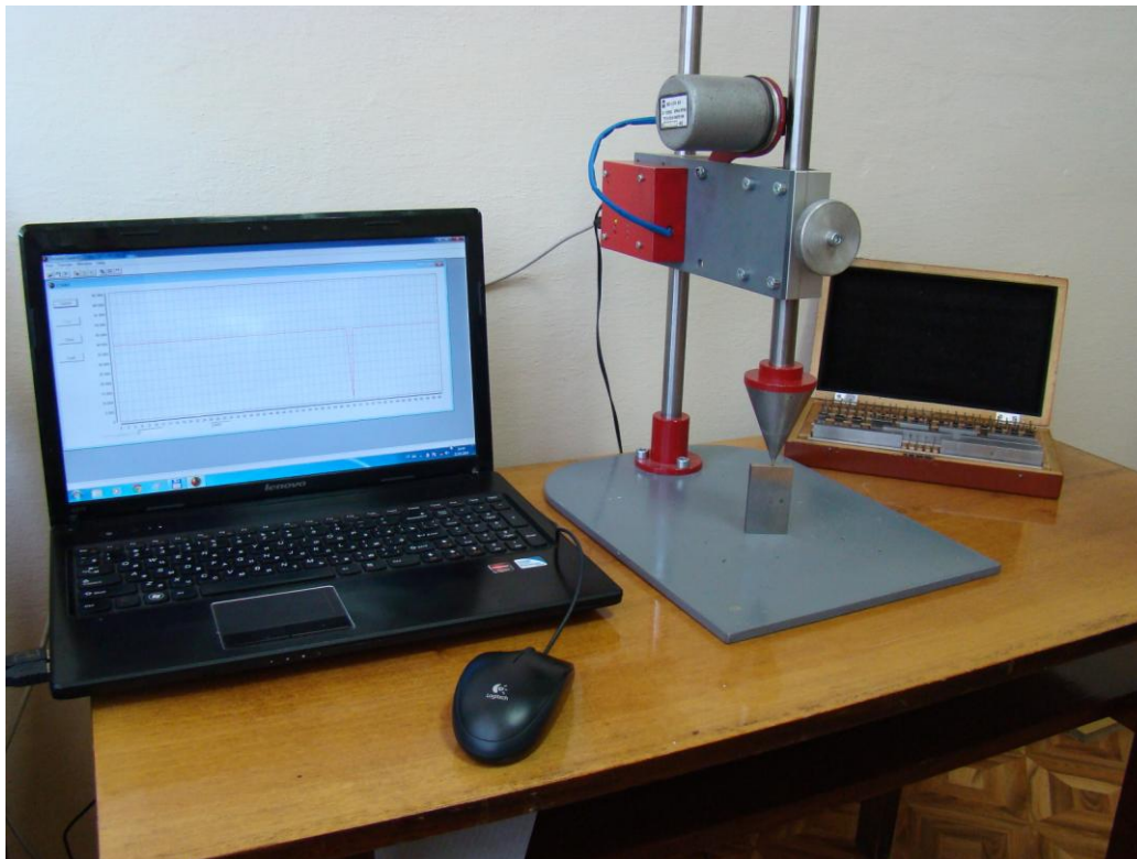
Рис. 1. Загальний вигляд інформаційно-виміральної системи
