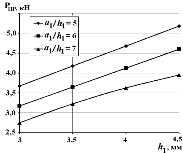
Рис. 6. Розрахунковий графік залежності необхідної для переміщення вершини різця на 0,3 мм сили приводу P_{\text{ПР}} від товщини h_1 і h_2 та довжини a_1 і a_4 пружних пластин
