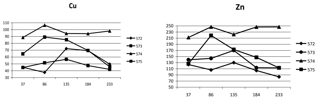
Рис. 2. Зміна вмісту хімічних елементів з глибиною для різних свердловин
