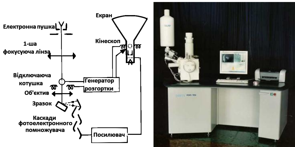
Рис. 1. Схема роботи растрового мікроскопа РЕМ-106І
