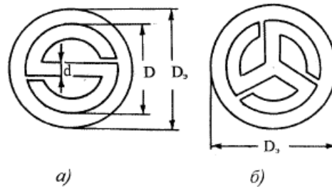
Рис. 9. Конструкція аплікаторної антени: а) двопрменевої, б) трипрменевої
