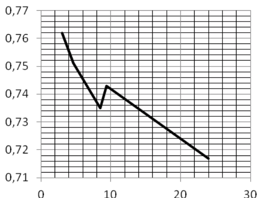
Рис. 3. Графік зміни дійсної частини коефіцієнта відбиття від частоти
