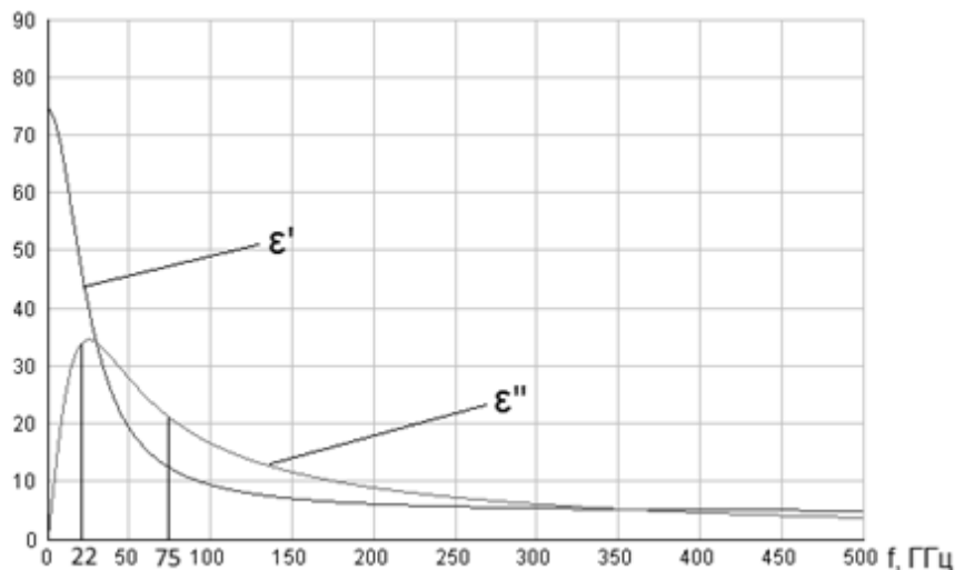
Рис. 1. Графік залежності діелектричної провідності води від частоти
