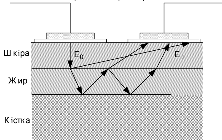
Рис. 7. Схема досліду з аплікаторною приймальною антеною
