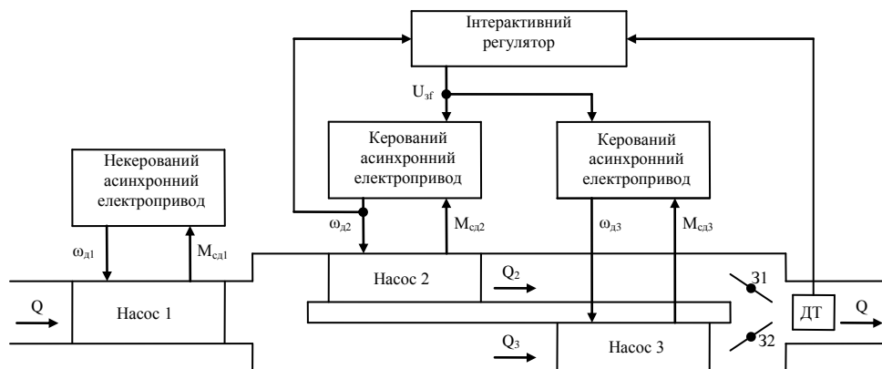
Рис. 2. Функціональна схема інтерактивної електро механічної системи
