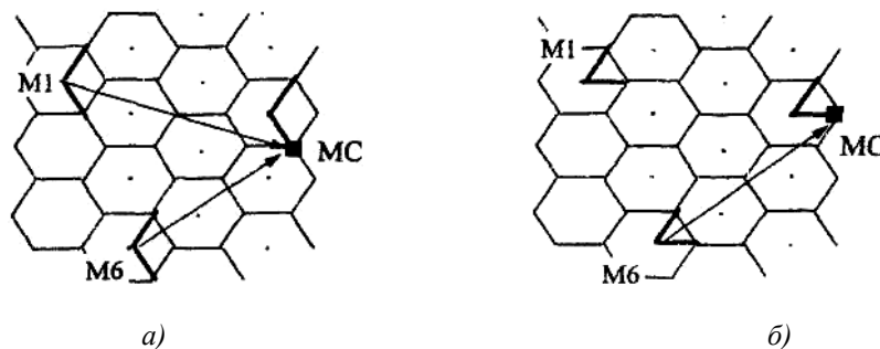
Рис. 2. Фрагменти ЧТП у разі N = 7 з використанням секторних антен з ШДС: а) \alpha = 120^\circ , б) \alpha = 60^\circ
