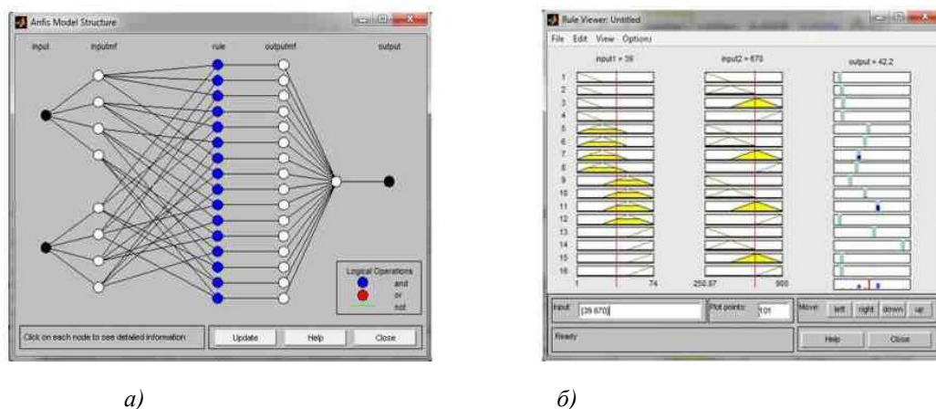
Рис. 4. Гібридна мережа: а – структура гібридної мережі, б – результат роботи експертної системи
