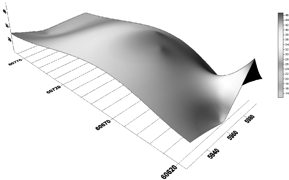
Рис. 4. Геометризація родовища габро за відносними площами рівномірного забарвлення
