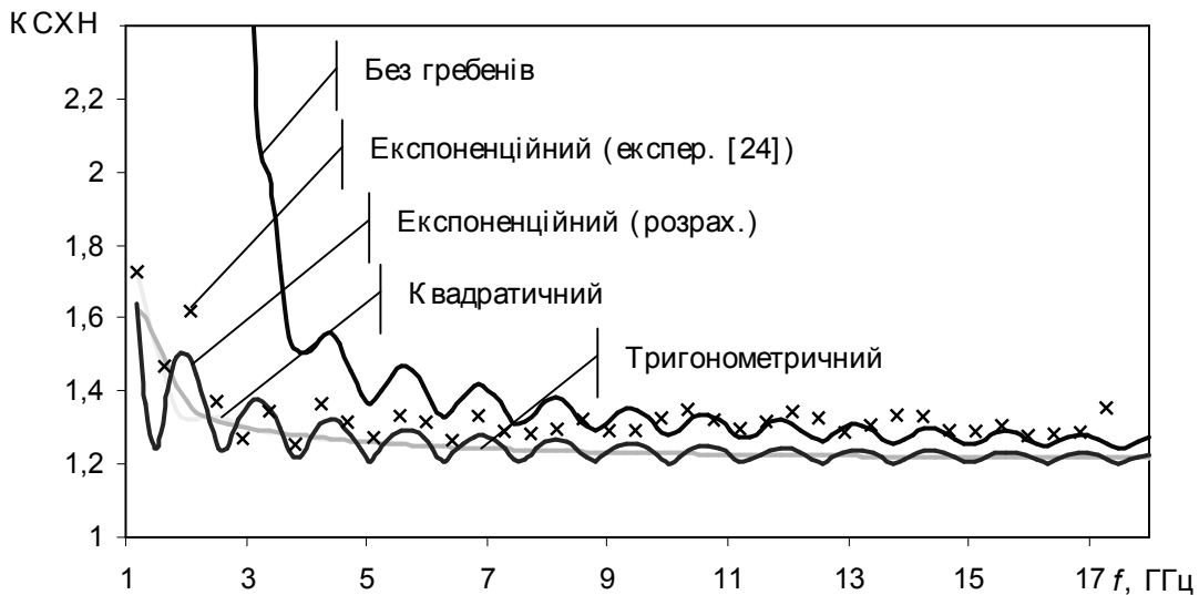
Рис. 3. Залежність КСХН від частоти широкосмугової рупорної антени на основі двогребеневого хвильоводу для різних законів зміни твірних розкриву
