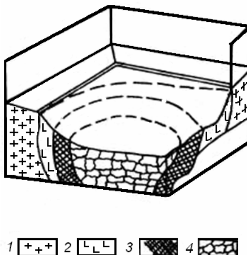
Рис. 1. Схема найбільш поширеної редькоподібної форми пегматитів Волинського родовища (вертикальний розріз), Вишняківська ділянка: 1 – біотито-амфіболітова зона; 2 – письмова (графічна) зона пегматиту; 3 – польовошпатована зона; 4 – кварцова зона
