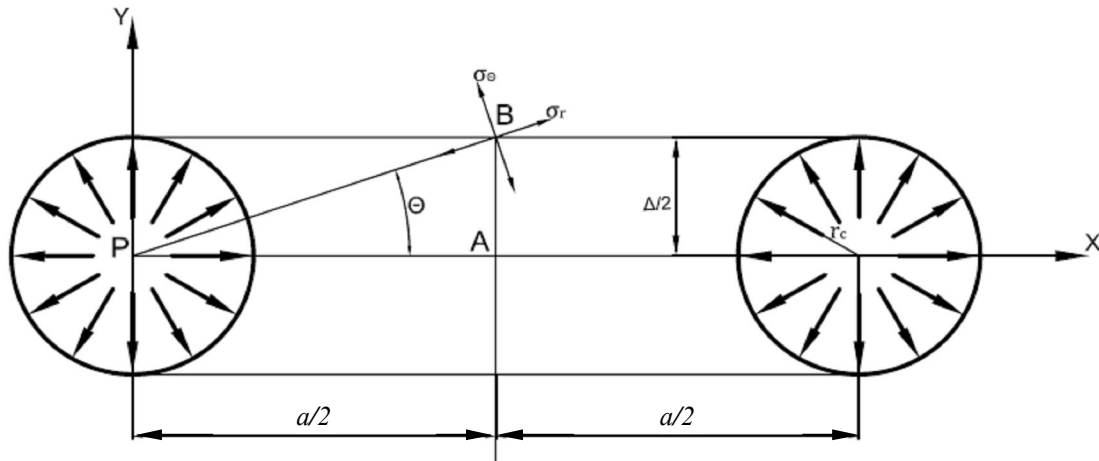
Рис. 1. Схема визначення параметрів контурного підривання
