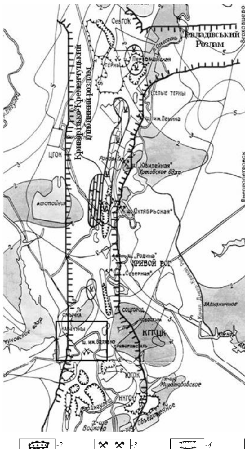
Рис. 1. Схема розташування глибинних розломів на території Криворізького басейну:
