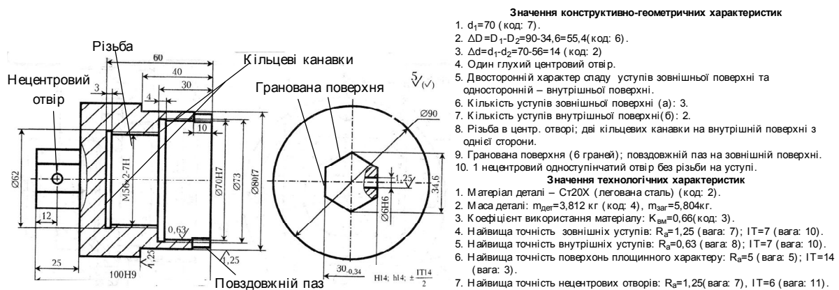
Рис. 4. Приклад деталі та значення конструктивно-геометричних та технологічних характеристик для її вхідного вектора НМ
