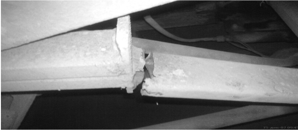
Рис. 2. Тріщини в горизонтальній частині об'ємного каркаса автобуса ЛАЗ-695НГ
