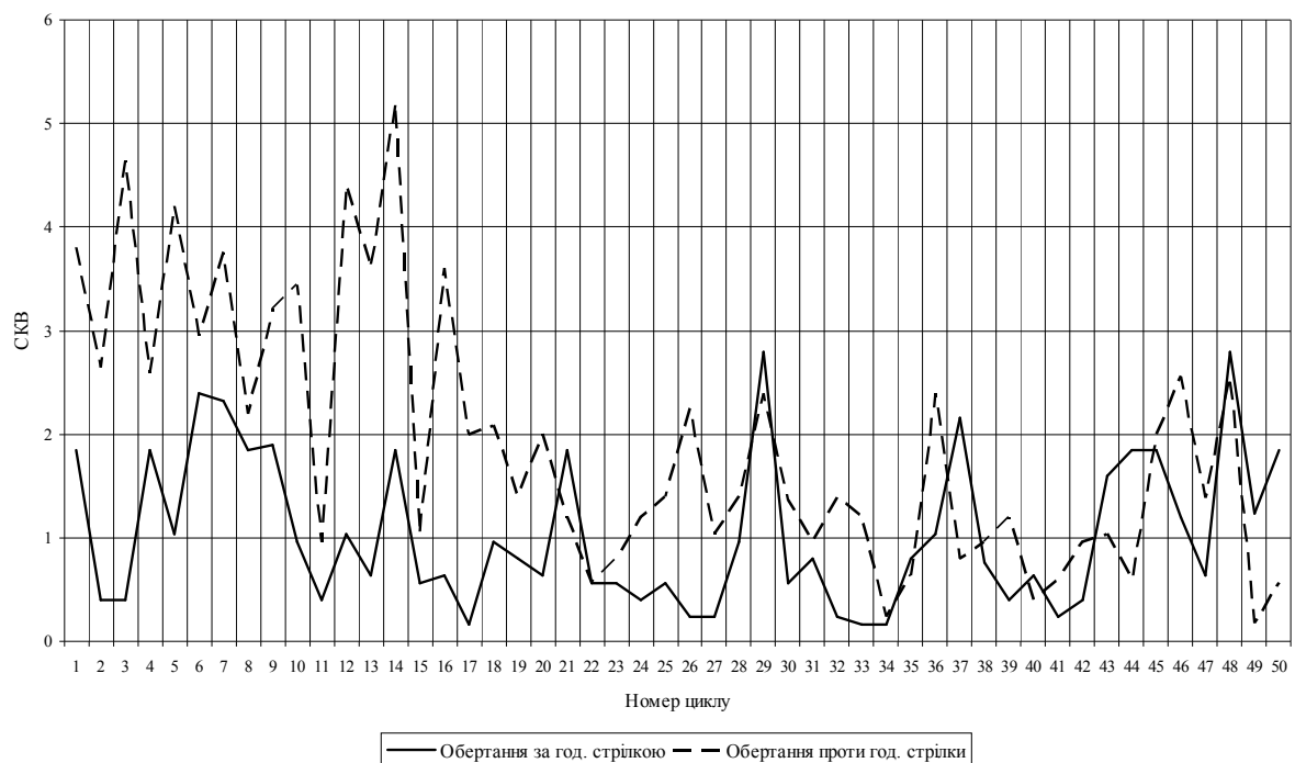
Рис. 4. СКВ для кожного виміряного півциклу
