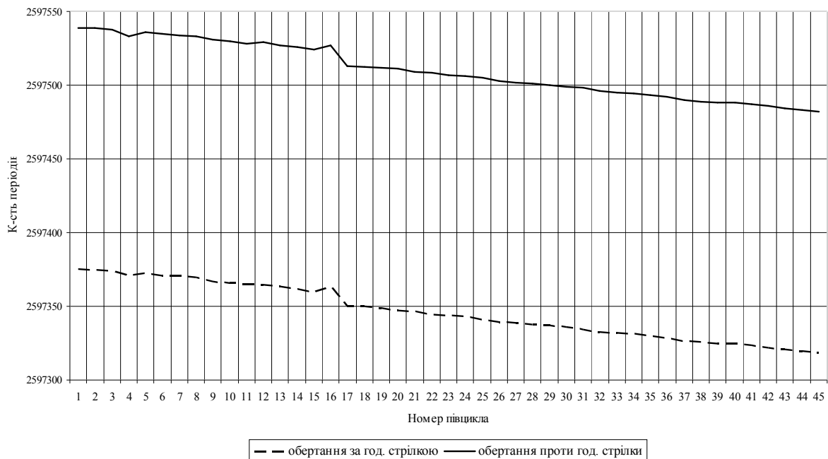
Рис. 1. Середнє значення \bar{N}_- та \bar{N}_+ , виміряних в одному циклі
